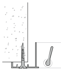
F1 – Parafuso
